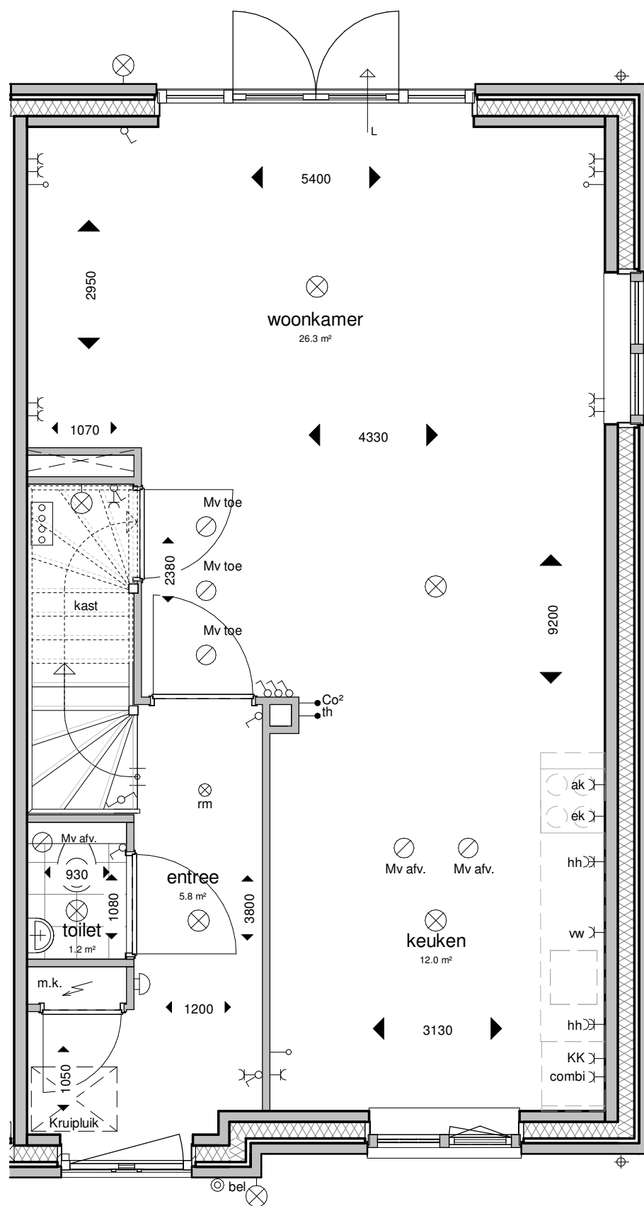
Begane grond
