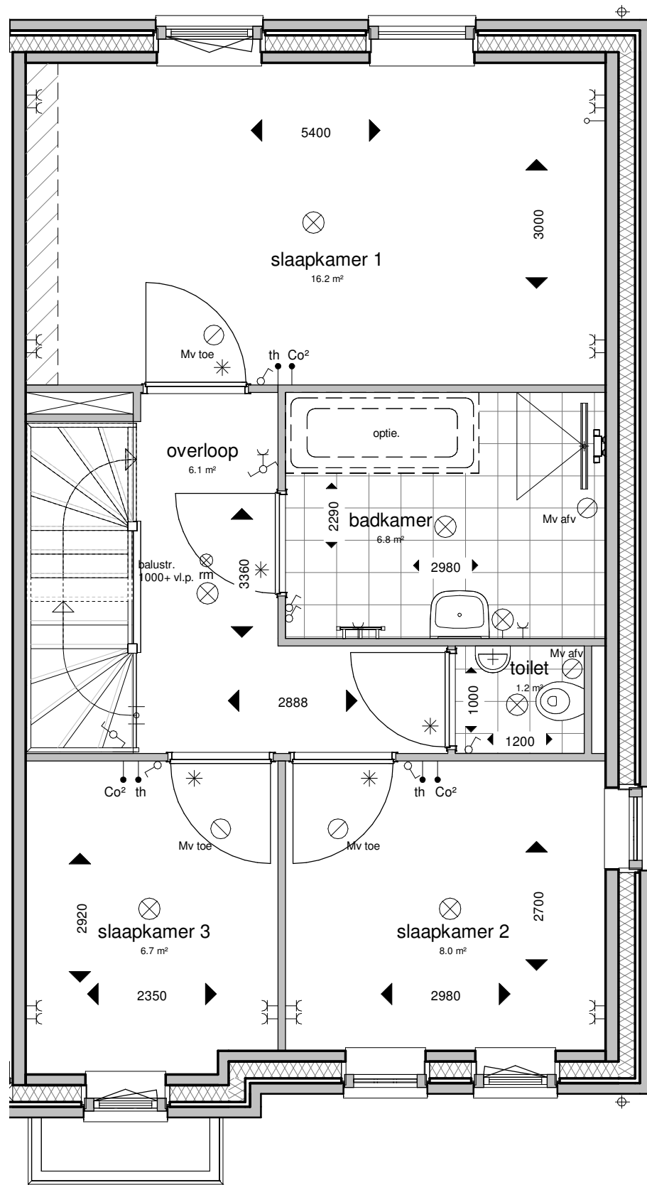
1e Verdieping
