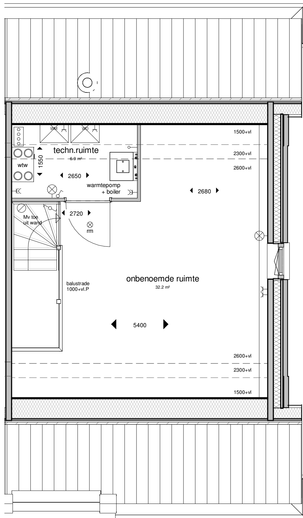
2e Verdieping
