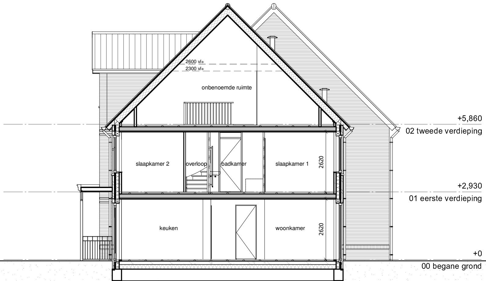
Doorsnede
