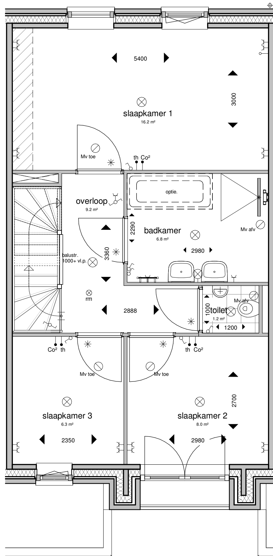
1e verdieping
