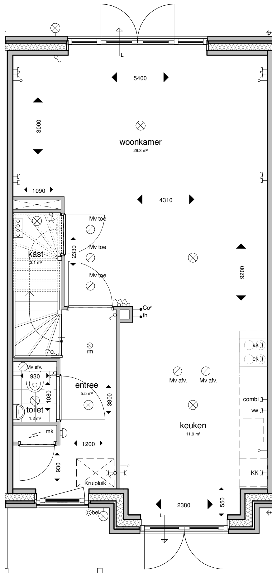
begane grond
